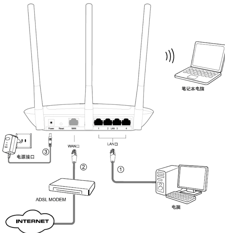
图 4-1 TL-WR886N 硬件安装示意图
